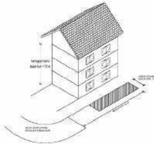
Gambar II. 35 Fungsi hunian yang memiliki ketinggian lebih dari 10 meter harus dilengkapi dengan akses yang diberi perkerasan dengan area operasional (bidang kerja) sekurang kurangnya memiliki lebar 4 meter dan panjang tidak melebihi 45 meter
