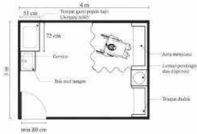
Gambar 11.192 Contoh desain ruang laktasi
