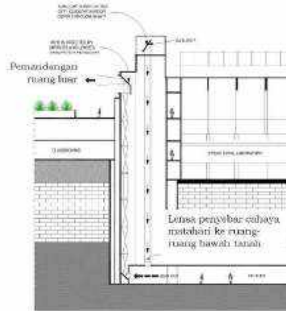
Gambar II.319 Contoh Penghadiran Pemandangan Luar ke Ruang Bawah (2/2)
