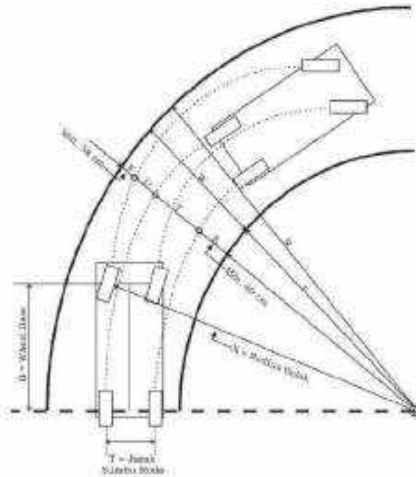
Gambar II.259 Prinsip dasar desain jalur mobil
