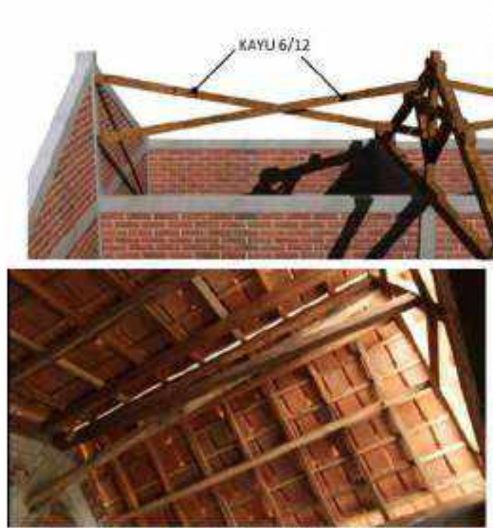
Gambar II.395 Ikatan Angin Antara Kuda-Kuda Kayu dengan Gunung-Gunung/ Angig
