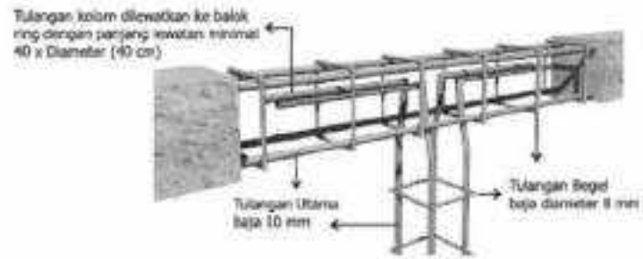
Gambar II.407 Hubungan Antar Kolom dengan Balok Keliling/ Ring
