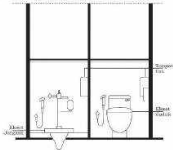
Gambar II.209. Potongan A toilet umum tipe moderat
