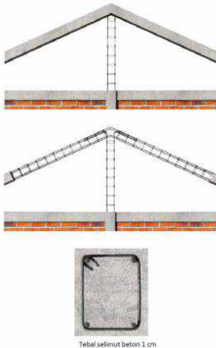
Gambar II.392 Tulangan Pada Bingkai Gunung-Gunung/ Ampir
