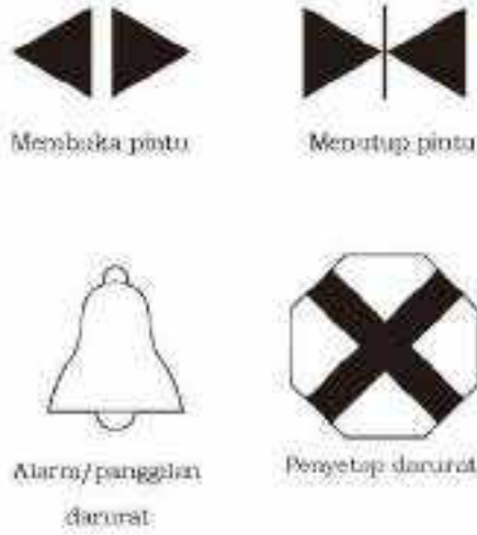
Gambar II.144. Standar symbol panel yang dibuat timbul
