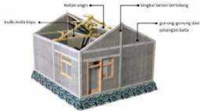
Gambar II.383 Struktur Atap
