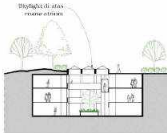
Gambar II.338 Contoh Bangunan Gedung di Bawah Tanah Yang Menggunakan Skylight (2/2)
