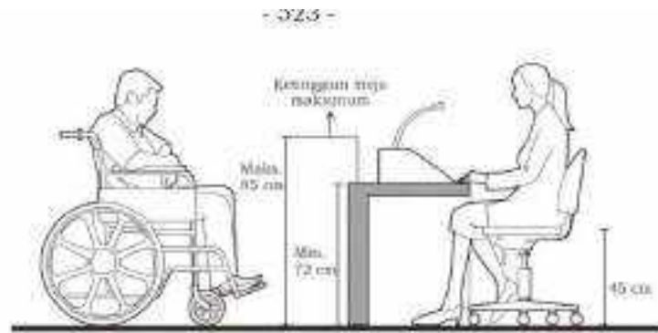
Gambar II.224. Dimensi meja pada pusat informasi tipe 1
