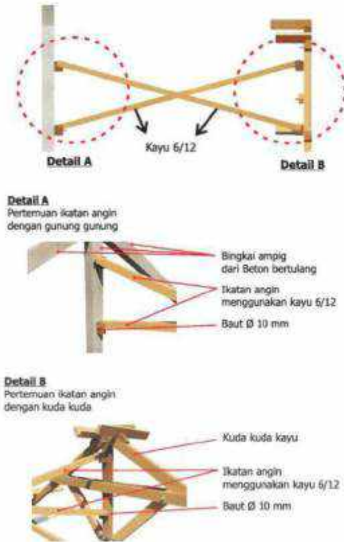
Gambar II.398 Detail Pertemuan Antara Ikatan Angin dengan Gunung-Gunung/Ampig
