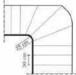
Gambar II.128. Contoh penerapan tangga kipas
