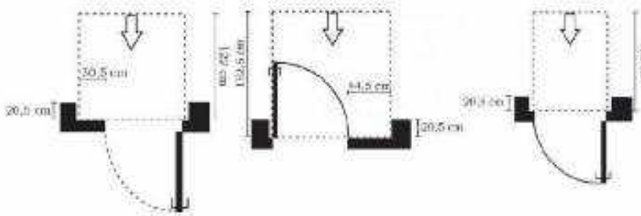
Gambar II.163. Ruang Bebas Pintu keluar
