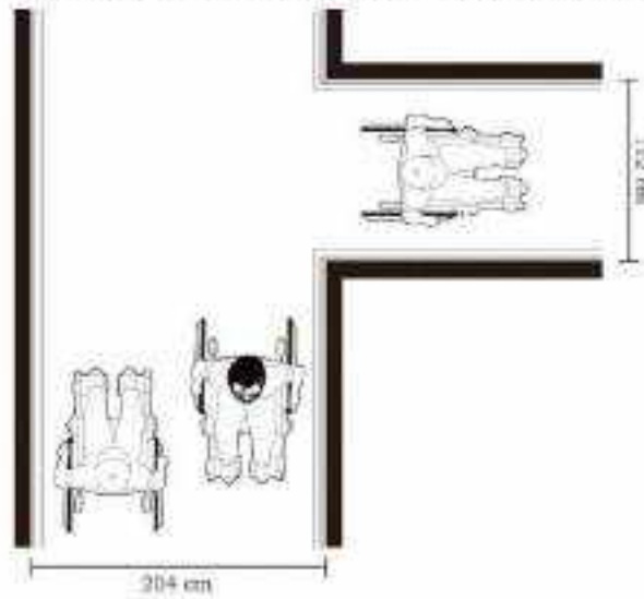
Gambar II.100. Lebar efektif koridor dengan pegangan ranzbol (handrail)
