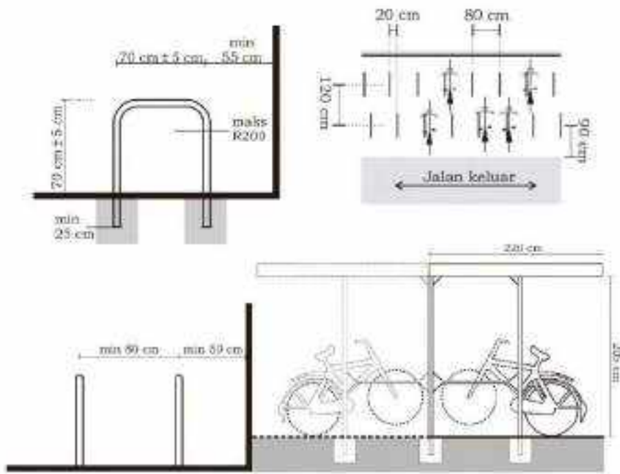
Gambar II.267 Ukuran dan contoh susunan tempat parkir sepeda
