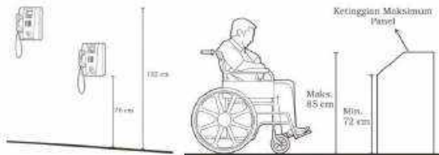
Gambar 3.43. Dimensi meja informasi dan perletakan telepon umum
