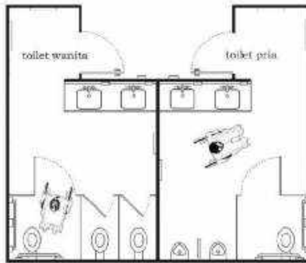
Gambar II.205. Contoh denah toilet yang setidaknya menyediakan 1 (satu) toilet penyandang disabilitas di toilet
