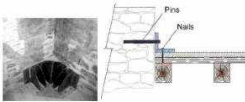
Gambar 11. 4 Penambahan Penghubung Antardinding dan Lantai di Sudut Ruang (kiri) dan Penambahan Pasak ( Pins ) dan Paku ( nails ) Penghubung di Sekeliling Antara Lantai Kayu dan Dinding Batuan (Kanan)
