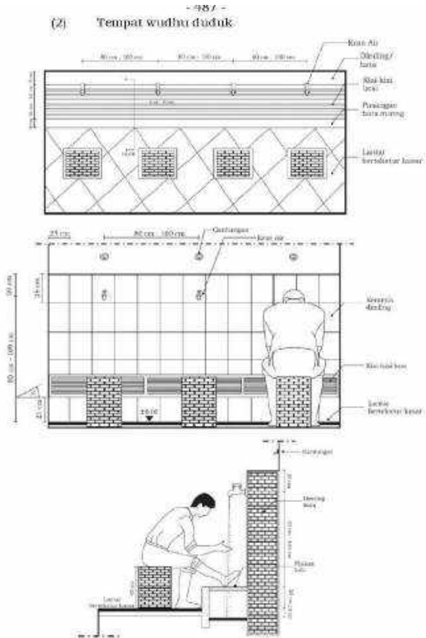
Gambar II.188. Dimensi tempat wudhu duduk (benah, tampak, dan potongan)
