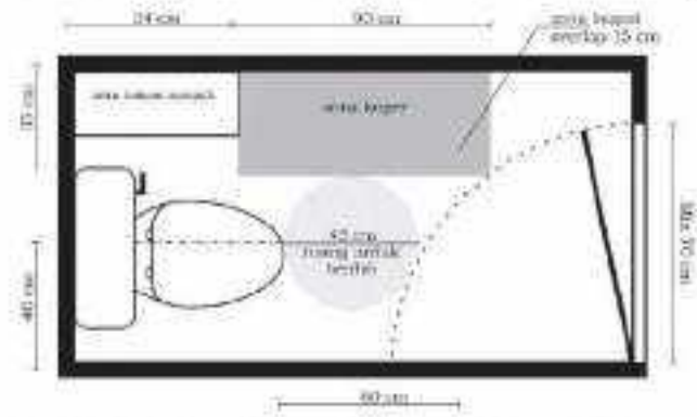
Gambar II.197. Ruang dalam toilet dengan bukaan ke dalam, tempat sampah, dan tempat berang bawahan.
