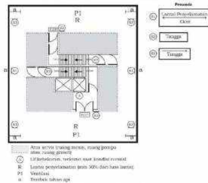
Gambar H.182. Ruang lantai penyelamatan
