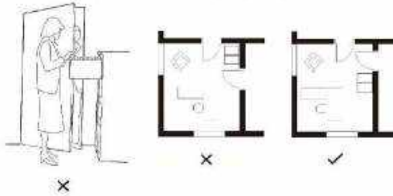
Gambar II.94. Penempatan perabot harus diberi jarak paling sedikit 75 cm dari bagian dalam pintu
