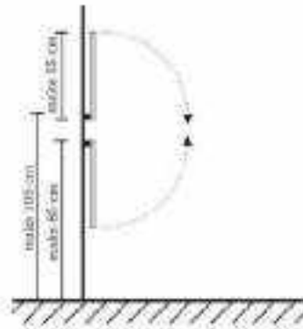
Gambar 11.193. Contoh desain tempat ganti popok bayi (changing table)
