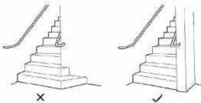
Gambar II.123. Akhir anak tangga yang menempel dengan dinding harus sejajar dengan dinding untuk mengurangi risiko kecelakaan
