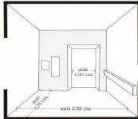
Gambar II.138. Detail ruang dalam lif penumpang
