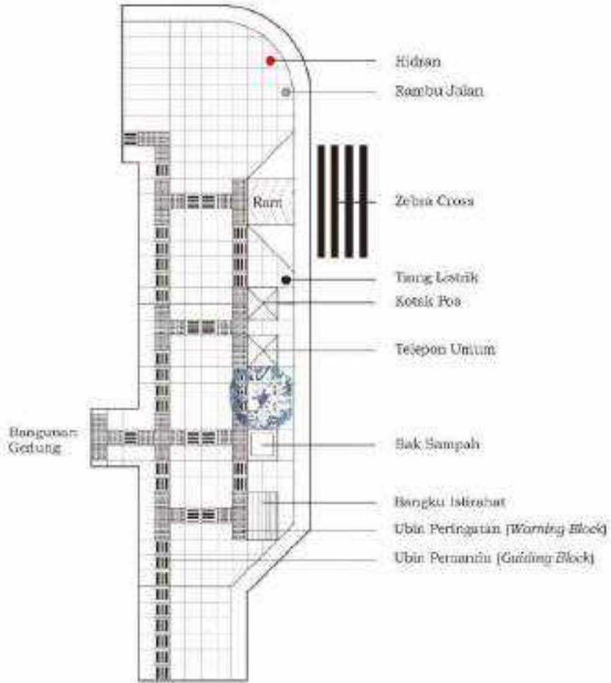
Gambar II.110. Prinsip perencanaan jalur pemacuda
