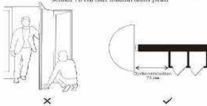
Gambar II.95. Pintu yang berdekatan (posisi buka) harus diberi jarak dan/atau tidak boleh membuka ke arah ruang yang sama
