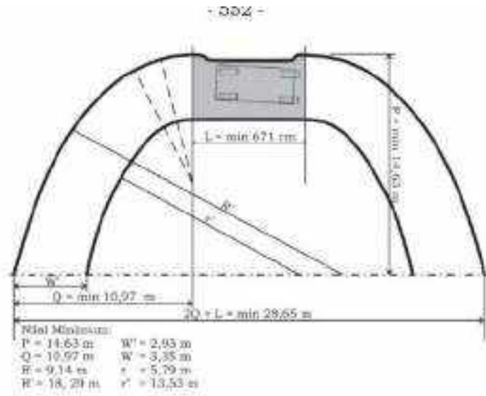
Gambar II.261 Dimensi kecilnya
