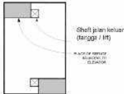
Gambar II.326 Contoh Kompartementalisasi Khusus
