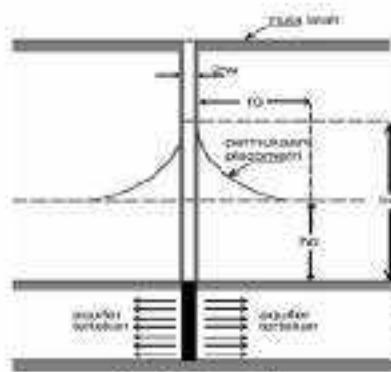
Aquifer tertekan
