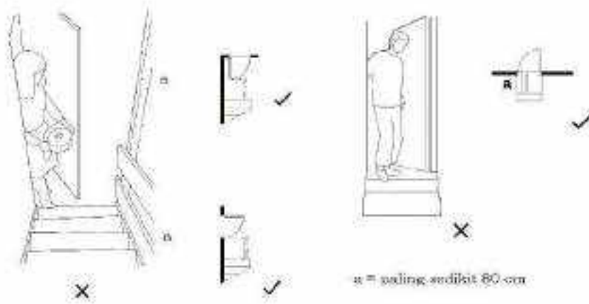
Gambar II.90. Pintu yang berdekatan atau berhadapan dengan tangga perlu diberi jarak
