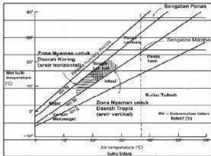
Gambar IV.2. Daerah Nyaman
