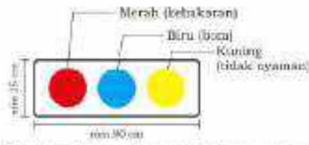
Gambar II.248. Alarm larangan darurat untuk pengunjung disabilitas ruang
