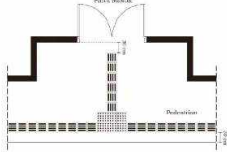
Gambar II.112. Contoh Penerapan Ubin Pemandu
