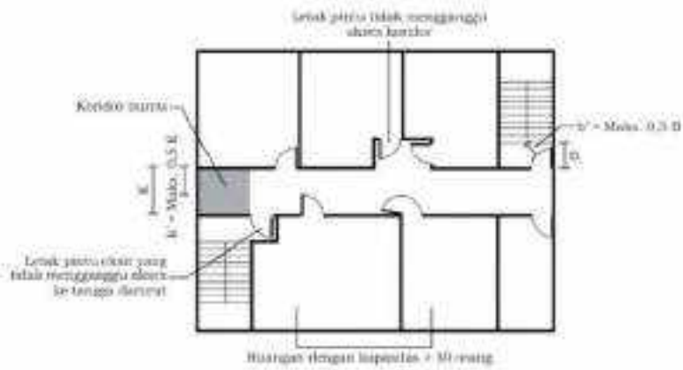
Gambar 2.80. Contoh penerapan akses eksit pada koridor buntu
