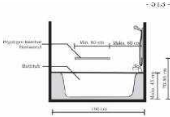
Gambar II.216. Dimensi bidet
