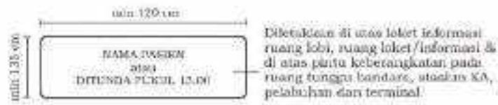
Gambar II.244. Fasilitas light sign (papan informasi) bagi penyandang disabilitas rambu
