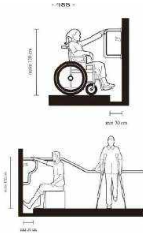
Gambar II.189. Dimensi tempat wadah duduk untuk penyandang disabilitas
