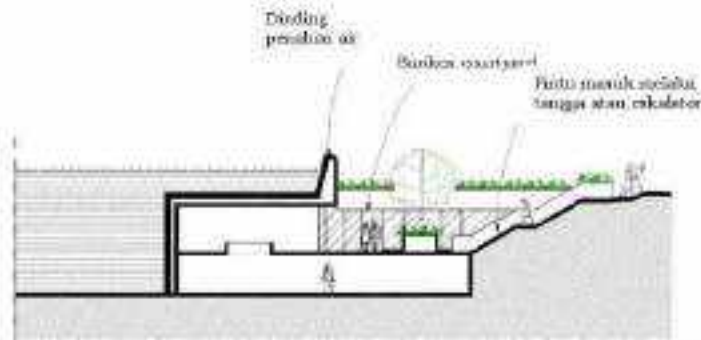
Gambar II.352 Contoh Jalan Masuk dan Keluar berupa Sunken Courtyard pada Bangunan Gedung di Bawah Air
