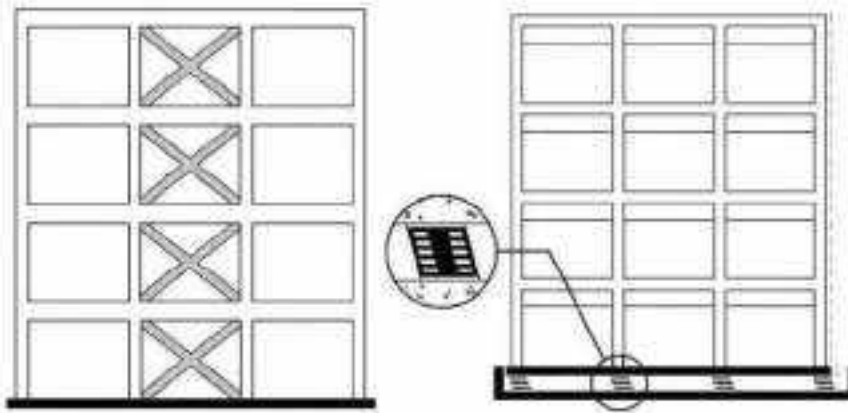
Gambar II. 3 Retrofitting dengan penambahan elemen diagonal (kiri) atau dengan menambahkan pengunci alas (kanan)
